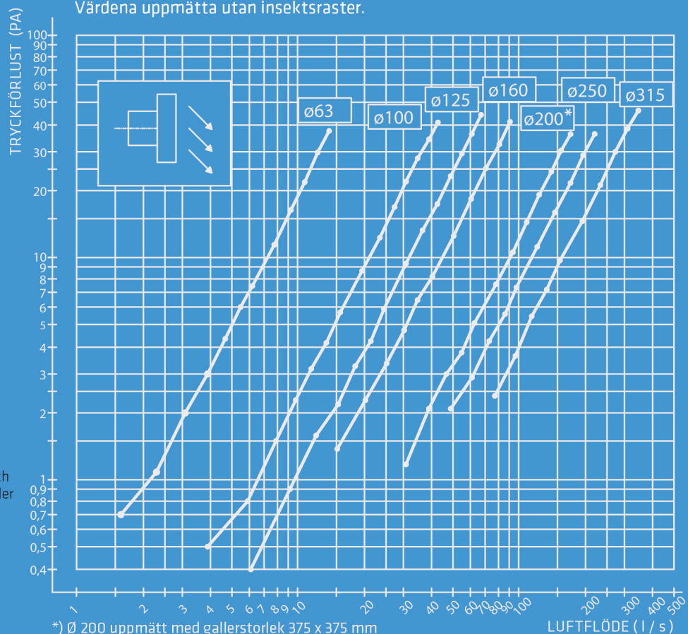
Maskinell luftväxling, avluft. Värdena uppmätta utan insektsraster.
