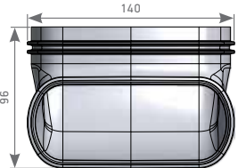
Вертикальный переходник 90°
