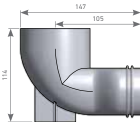
Горизонтальный переходник 90°
