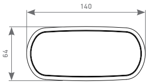
Полужесткий воздуховод
